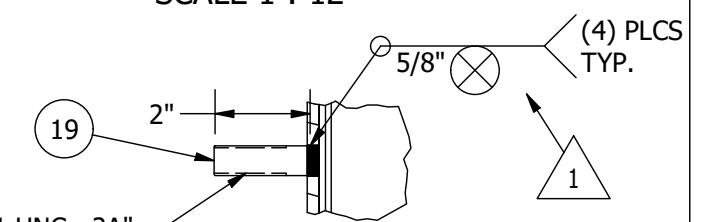
DETAIL WELD STUD
